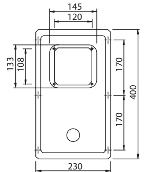
Kit pannello di chiusura per condotto fumi
